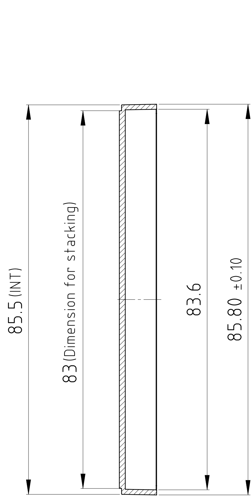
SECTION A-A
